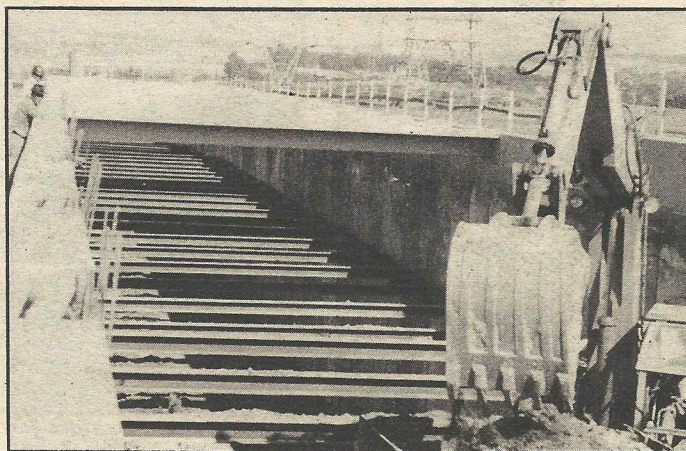
A cobertura, ao nível do solo, esconde a profundidade da trincheira
